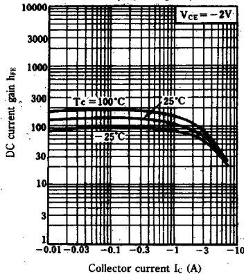
h_{FE} - I_C
