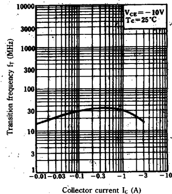
f_T - I_C
