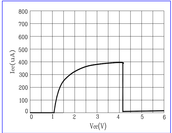
Fig. 2 I_{CC} - V_{CC}
