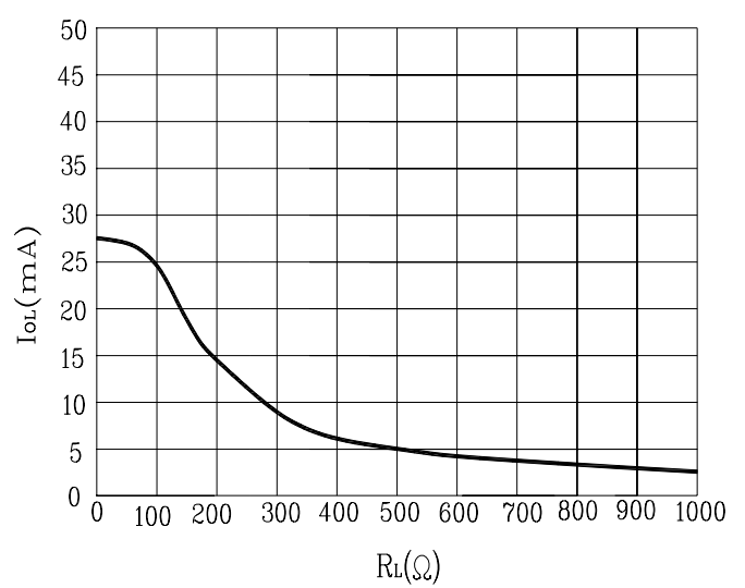
Fig. 4 I_{OL} - R_L
