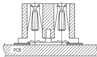
PCB ASS'Y
