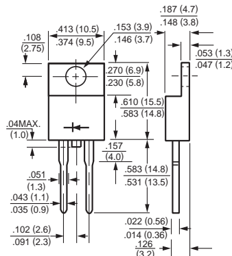
TO-220A
