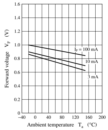
V_F - T_a
