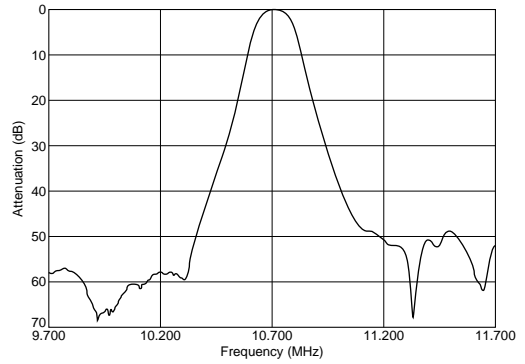
SFECV10M7JA00-R0
