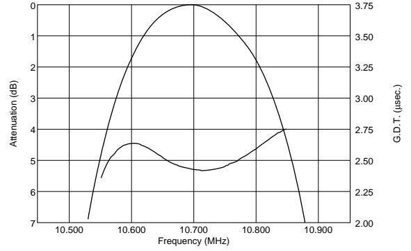
SFELA10M7GALP03-B0
