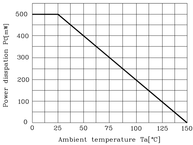
Fig. 3. P_d - T_a
