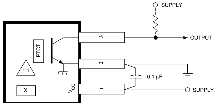
Dwg. EH-013
