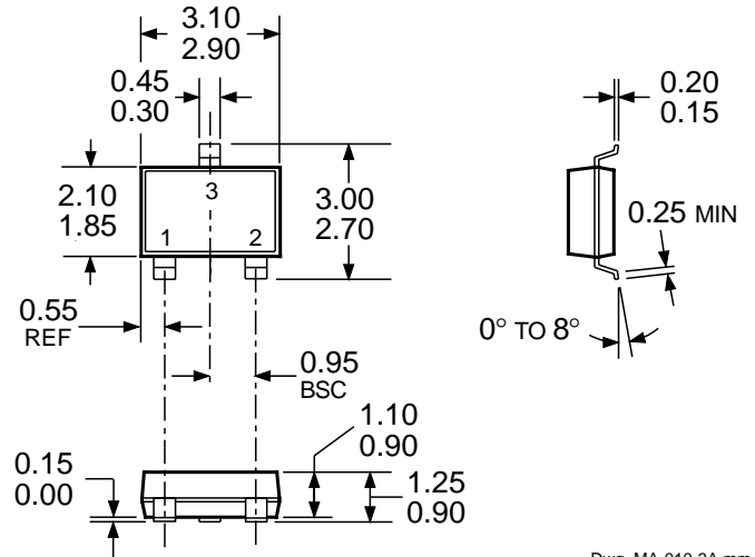
Dwg. MA-010-3A mm
