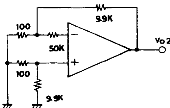
(4) I_B (+)
