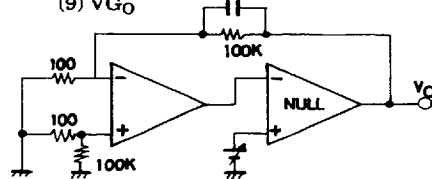
(9) V_{GO}
