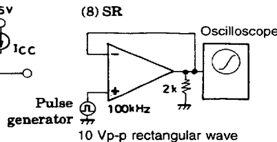
(8) SR
