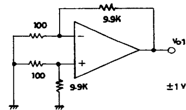
(1) V_{IO} , SVRR
