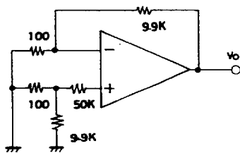
(5) I_B (-)
