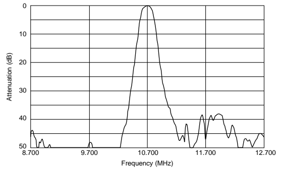
SF ECS10M7GA00-R0
