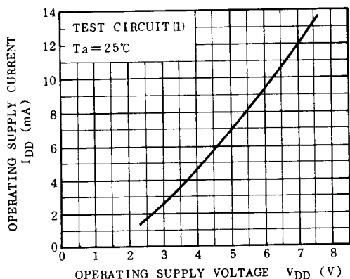
V_{DD} - I_{DD}
