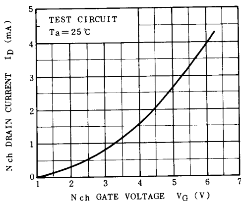
V_G - I_D
