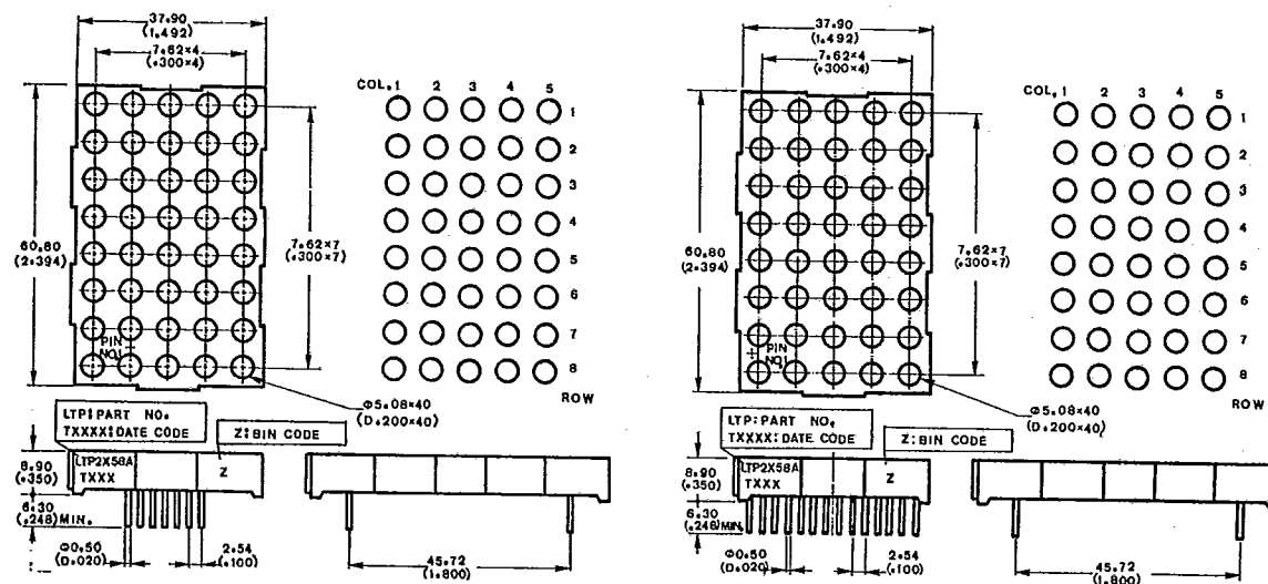
B. LTP-2458AA/2558AA
