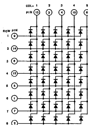
B. LTP-2158A
