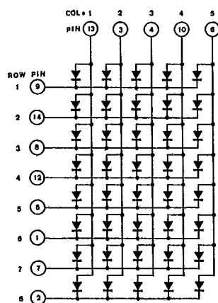
A. LTP-2058A
