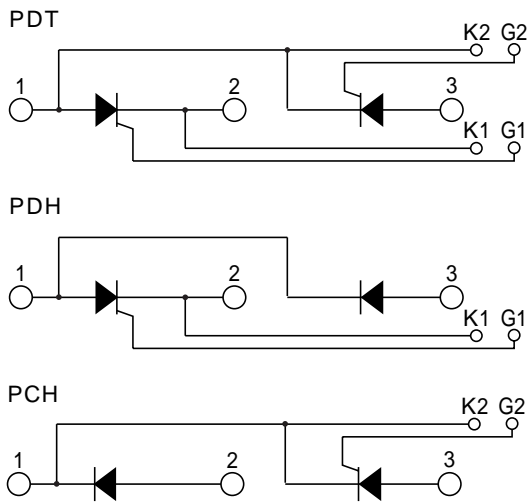
回路図 CIRCUIT
